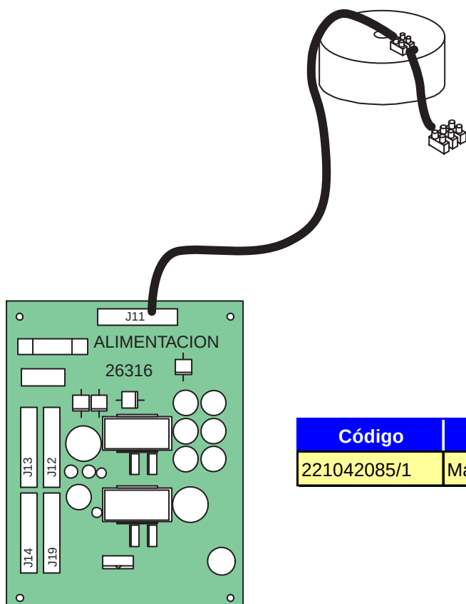
TRANSFORMADOR
