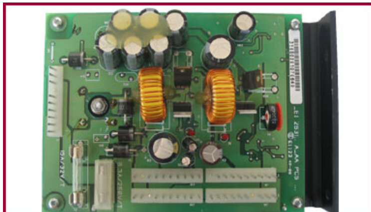
64801354/1 Fuente alimentación 26316
