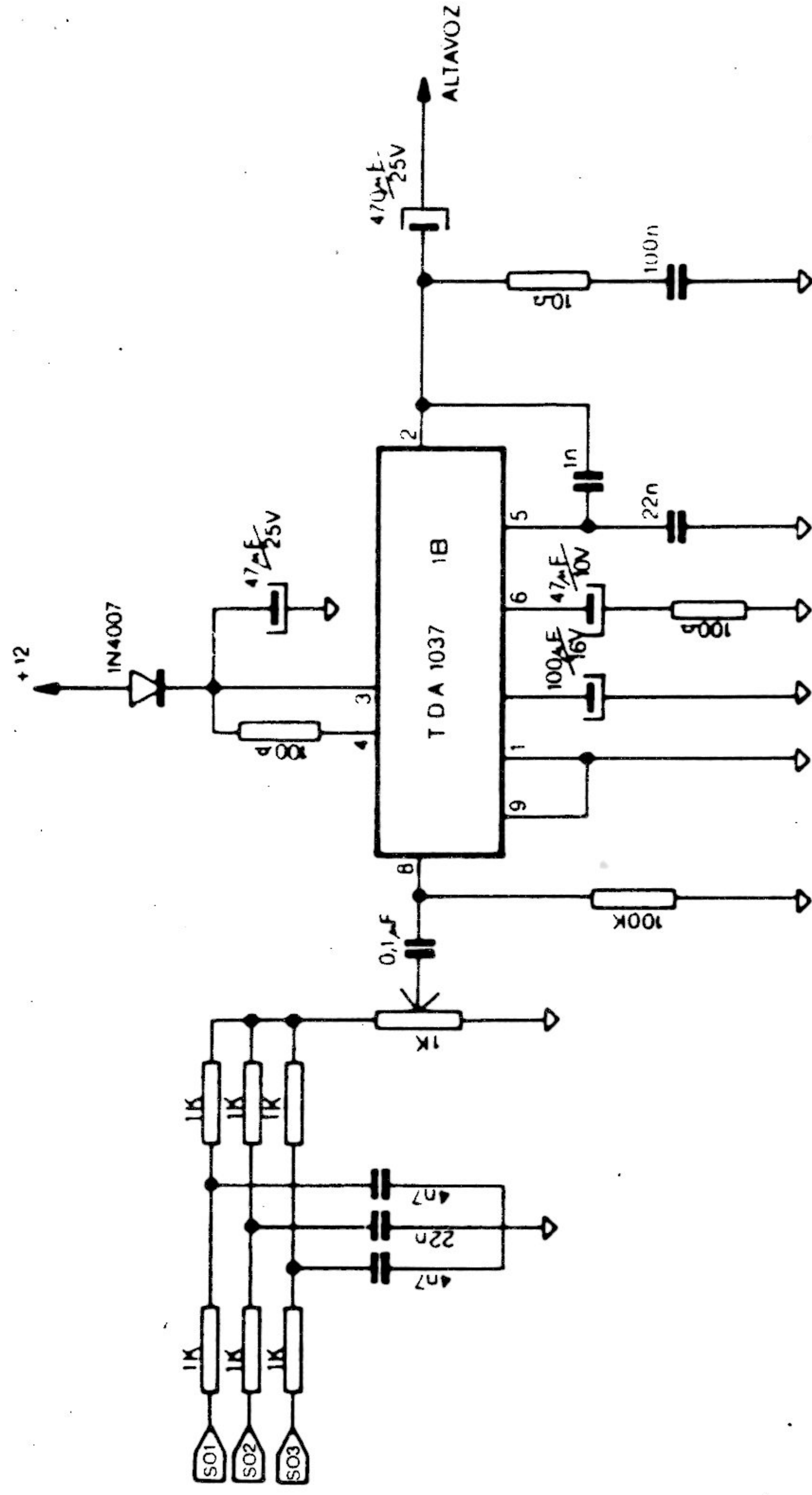
AMPLIFICADOR DE AUDIO
