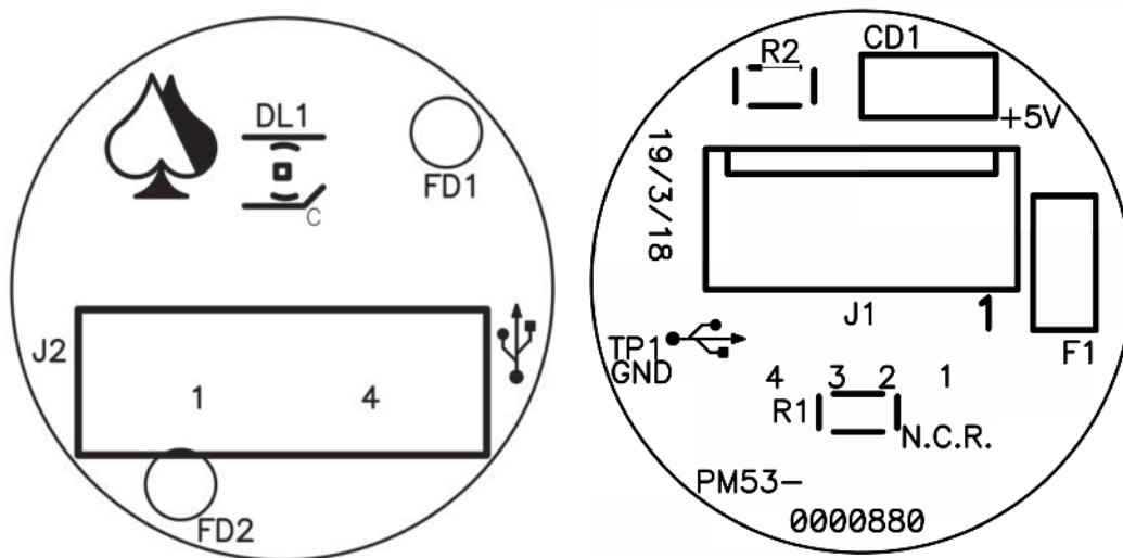
Serigrafía de Componentes
