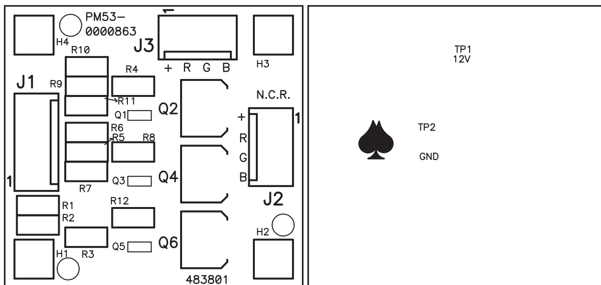
Serigrafía de Componentes
