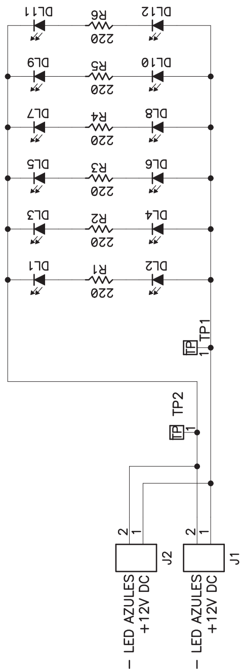
Serigrafía de Componentes
