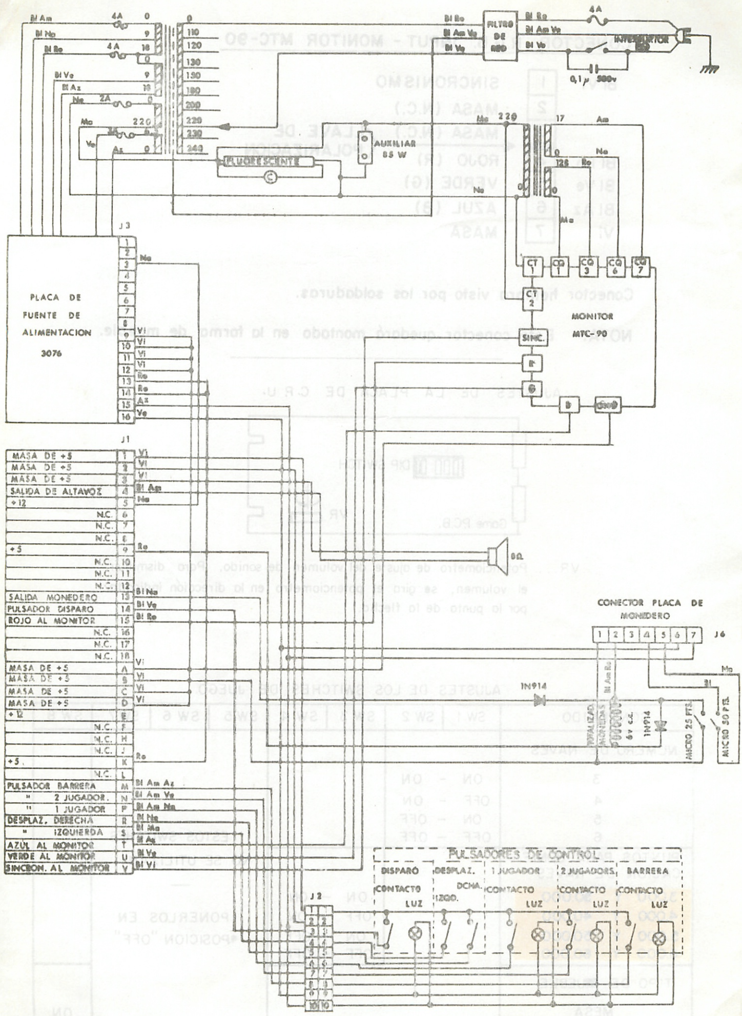
CABLEADO GENERAL PHOENIX RECREATIVOS FRANCO, S.A.
