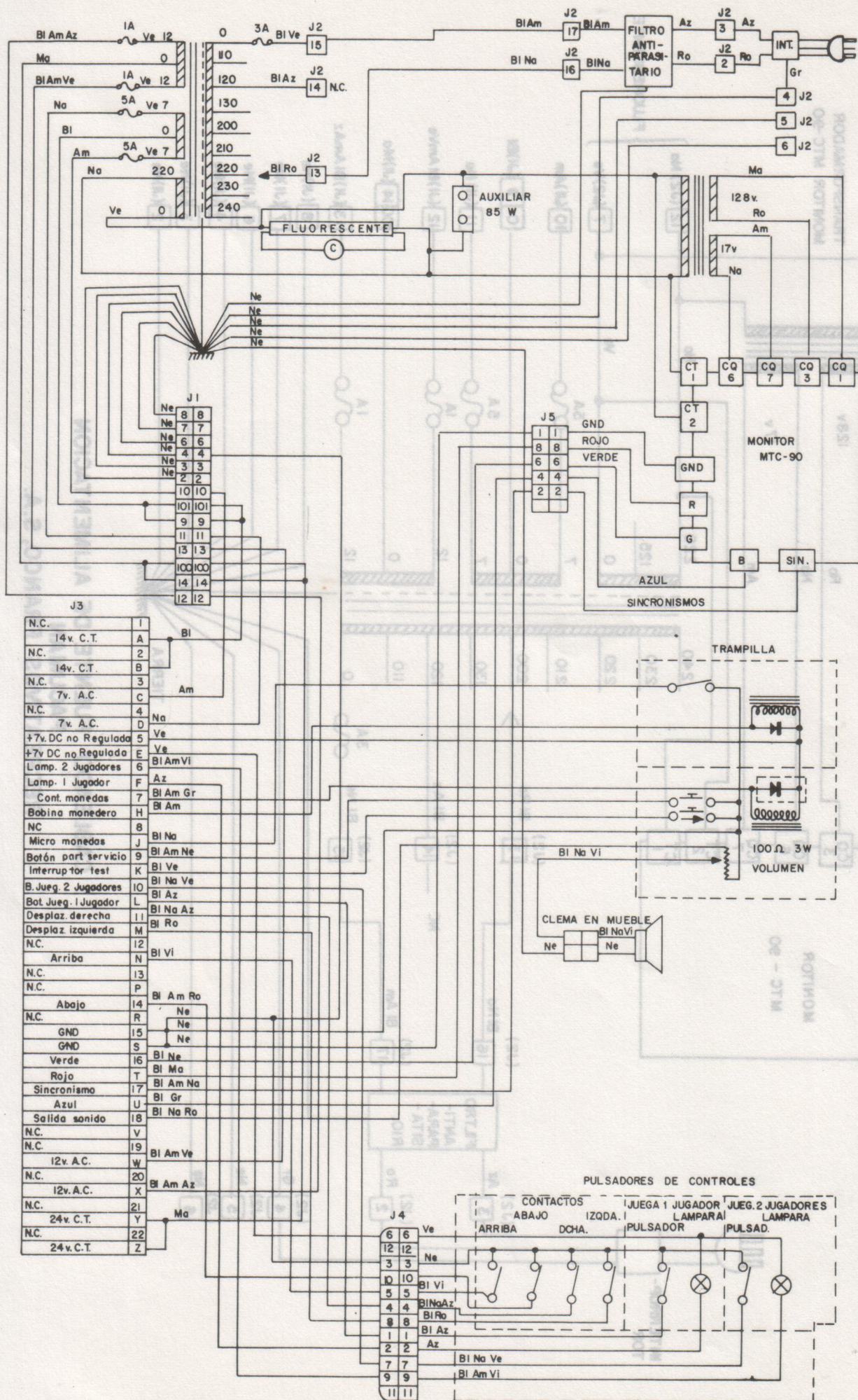
CABLEADO GENERAL PACUMAN RECREATIVOS FRANCO, S.A.
